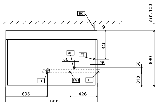
Boven aanzicht
